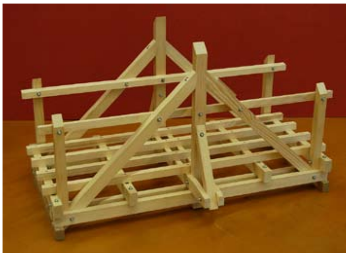
Brücken-Konstruktion
